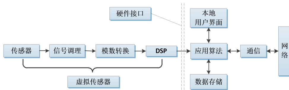
图 3.3.9 智能传感器一般模型
